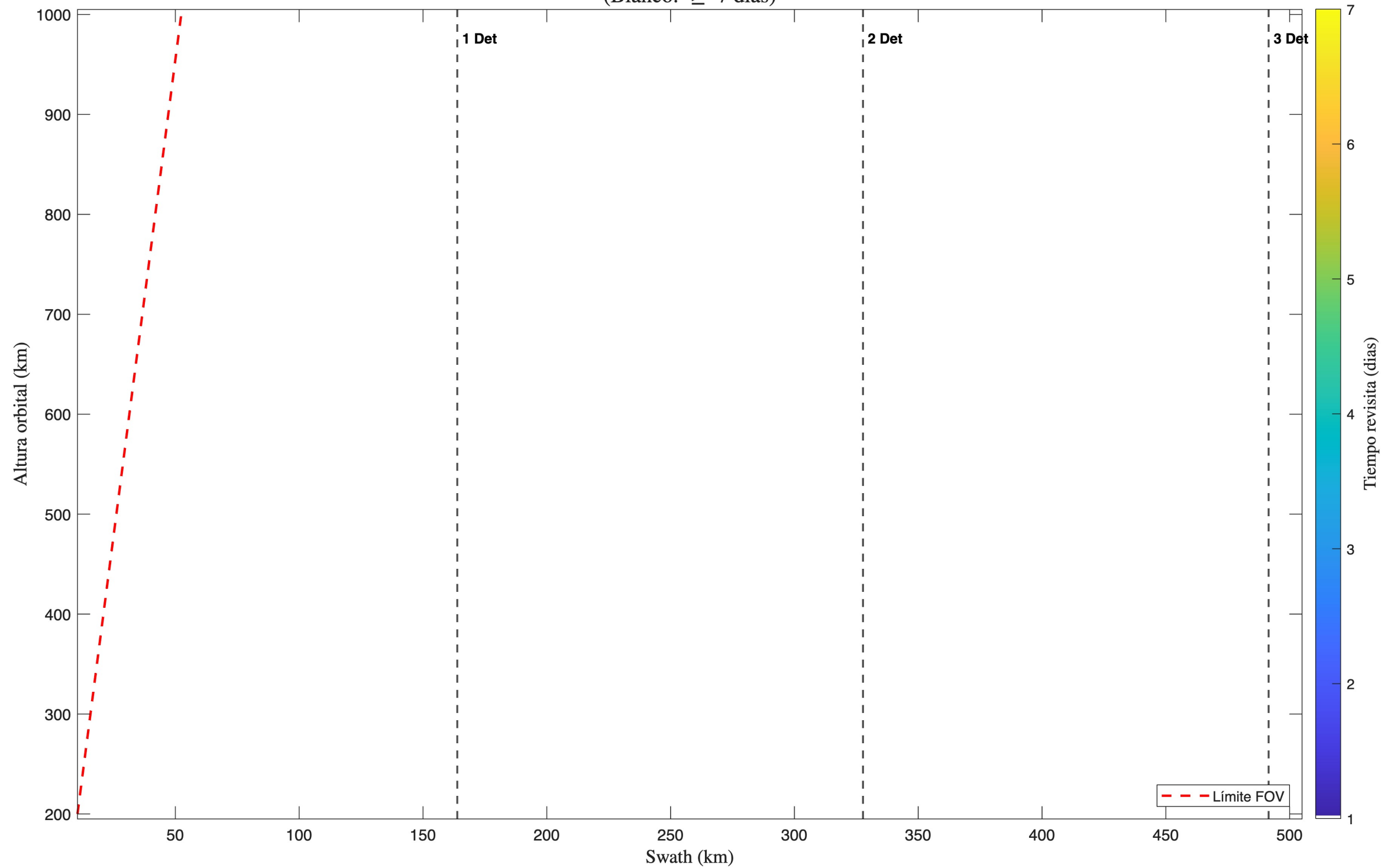
Tiempo Revisita - 2 Satellite(s); 1 Telescopio(s): Cassegrain; Detector 2 (Blanco: \geq 7 días)
